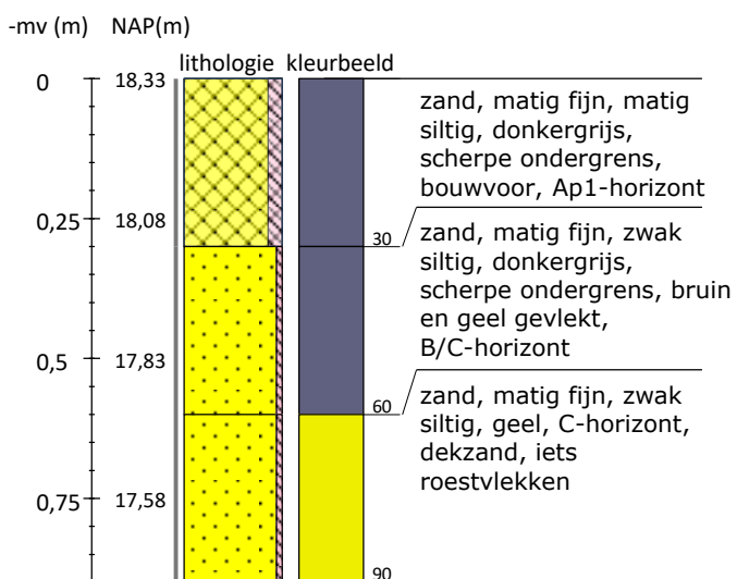
Boring 11 RD-coördinaten: 172711/468939
