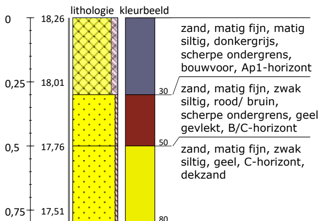
Boring 10 RD-coördinaten: 172680/468913
