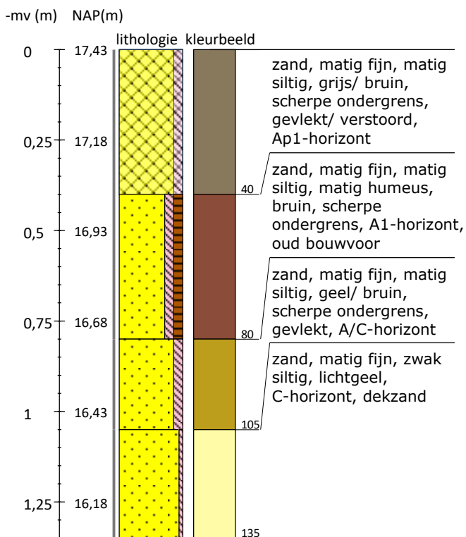
Boring 3 RD-coördinaten: 172472/468710
