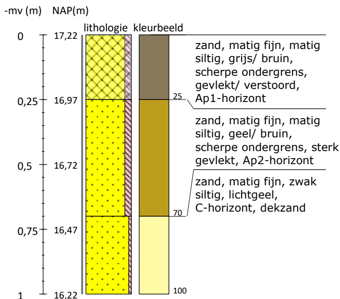
Boring 4 RD-coördinaten: 172532/468738
