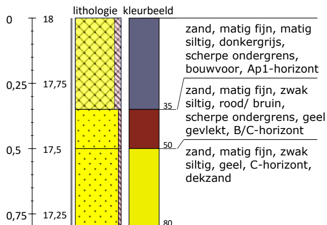
Boring 9 RD-coördinaten: 172710/468873
