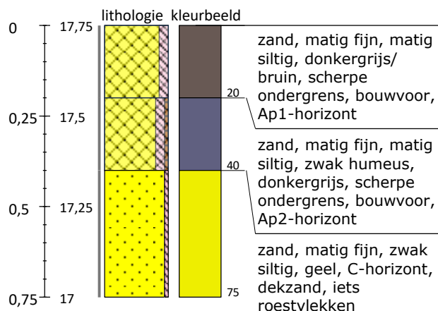
Boring 7 RD-coördinaten: 172617/468788
