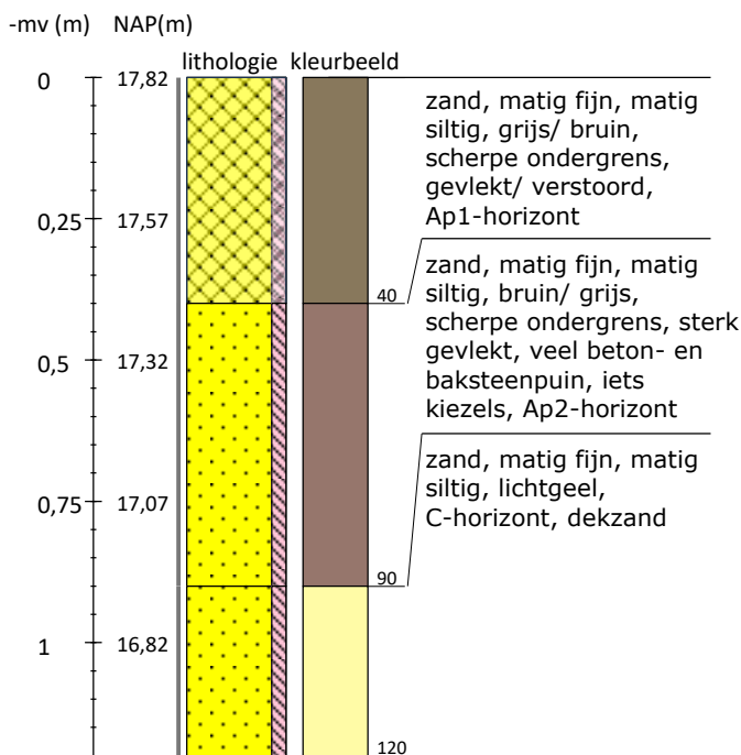
Boring 4 RD-coördinaten: 172532/468738
