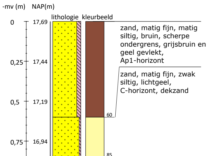
Boring 5 RD-coördinaten: 172569/468721
