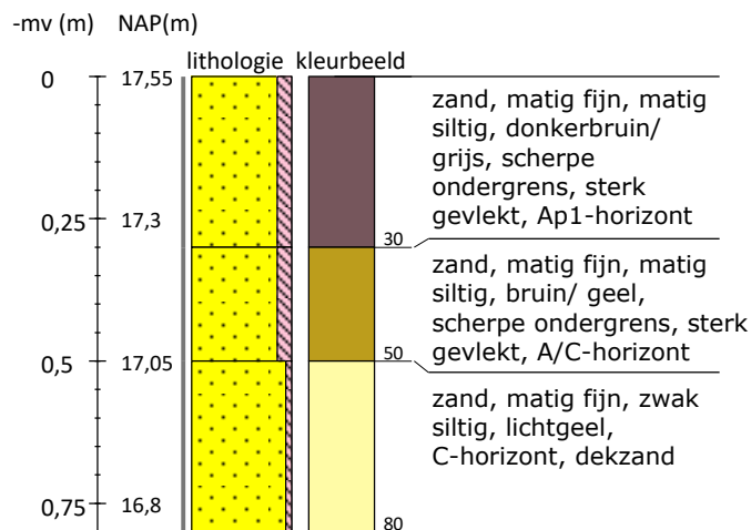
Boring 1 RD-coördinaten: 172439/468686
