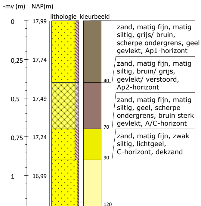
Boring 6 RD-coördinaten: 172608/468730
